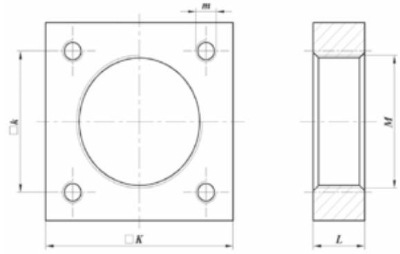
KARE CETOP FLANŞLARI
