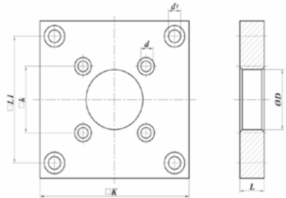
KARE CETOP ÖN BAĞLANTI FLANŞI
